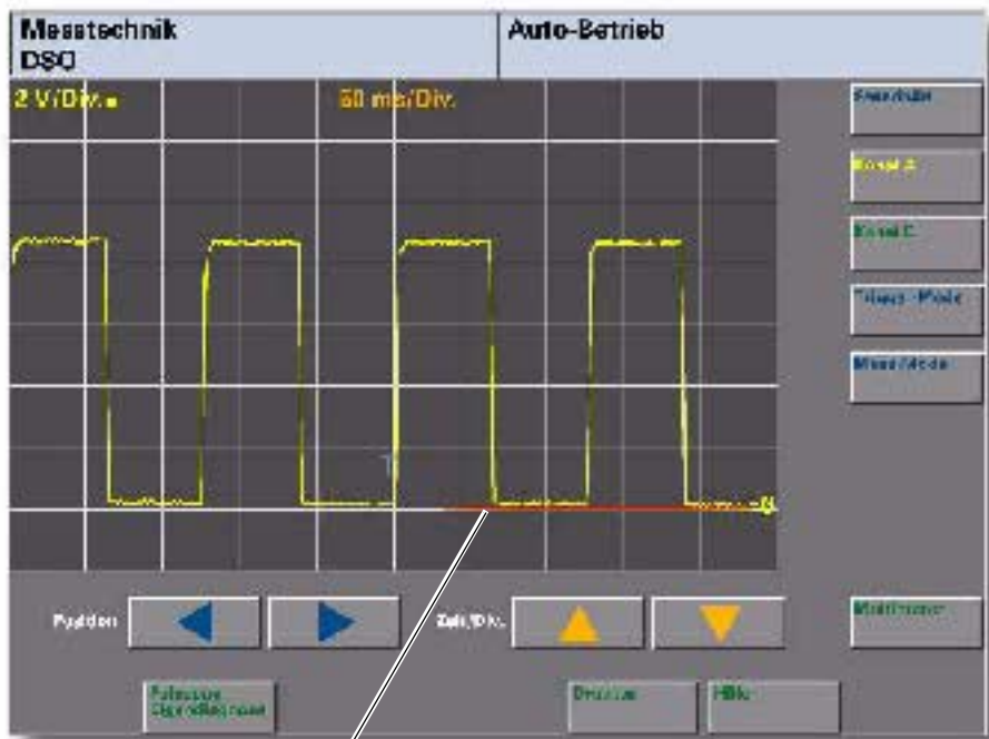
Уровень напряжения при скорости v = 0 км/ч
