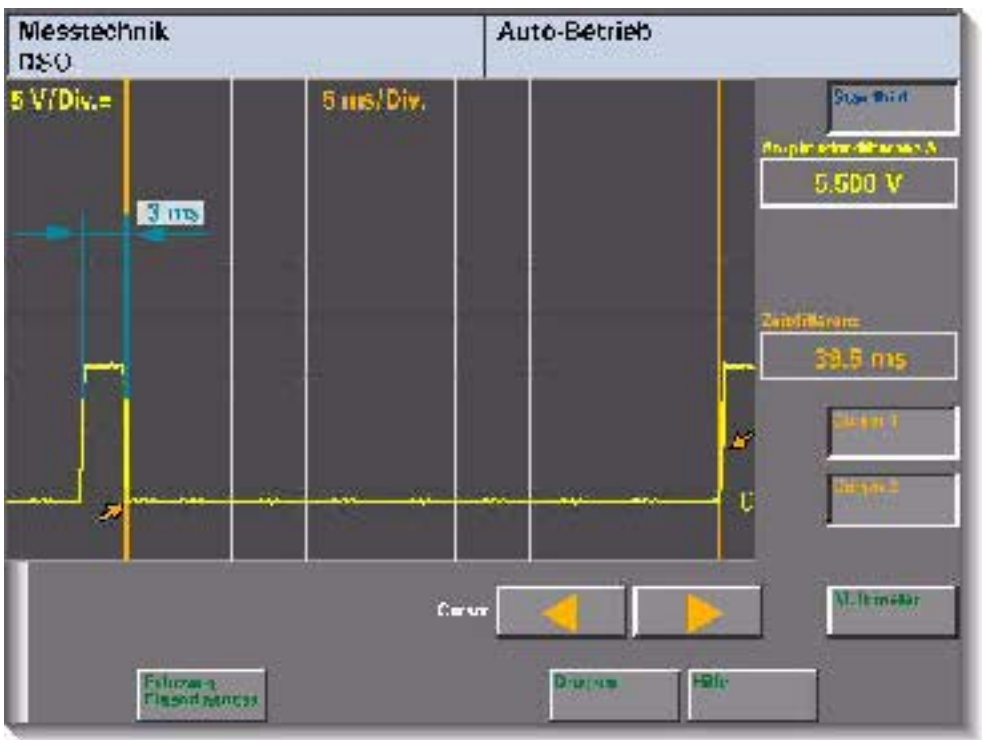
Изображение на экране DSO – сигнал от F189, селектор в положениях P, R, N, D или S
