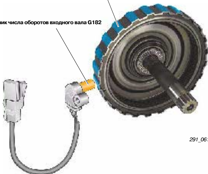
Держатель наружных дисков фрикциона K2 (зубчатое колесо для работы датчика G182)
