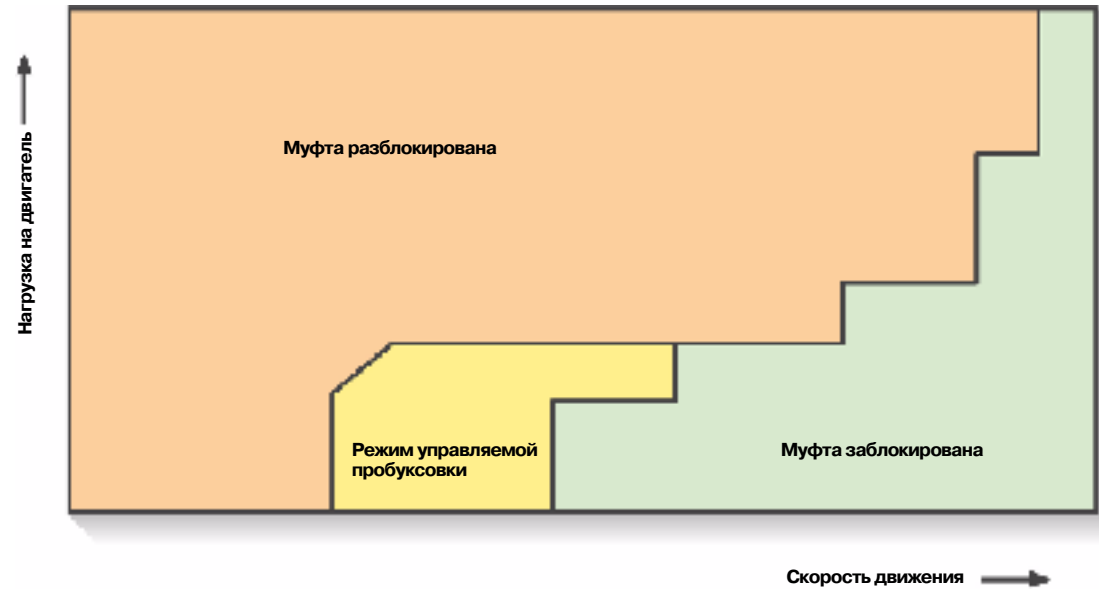
Муфта блокировки гидротрансформатора — селектор в положении «D»
