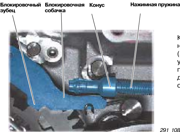
Положение «Нажимная пружина сжата»
