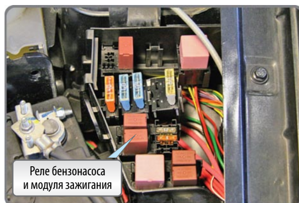
Фото 18.2. Реле бензонасоса и модуля зажигания
