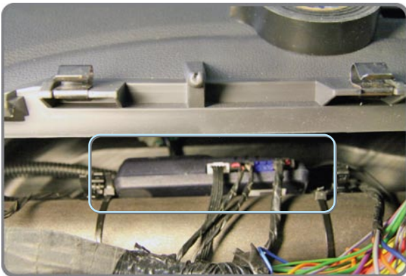
Фото 8. Блок сигнализации
